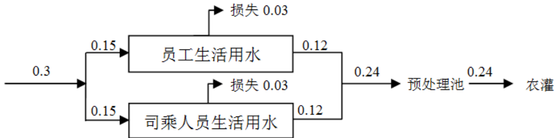
图 2-1 项目水平衡图（消耗单位：m 3 /d）
