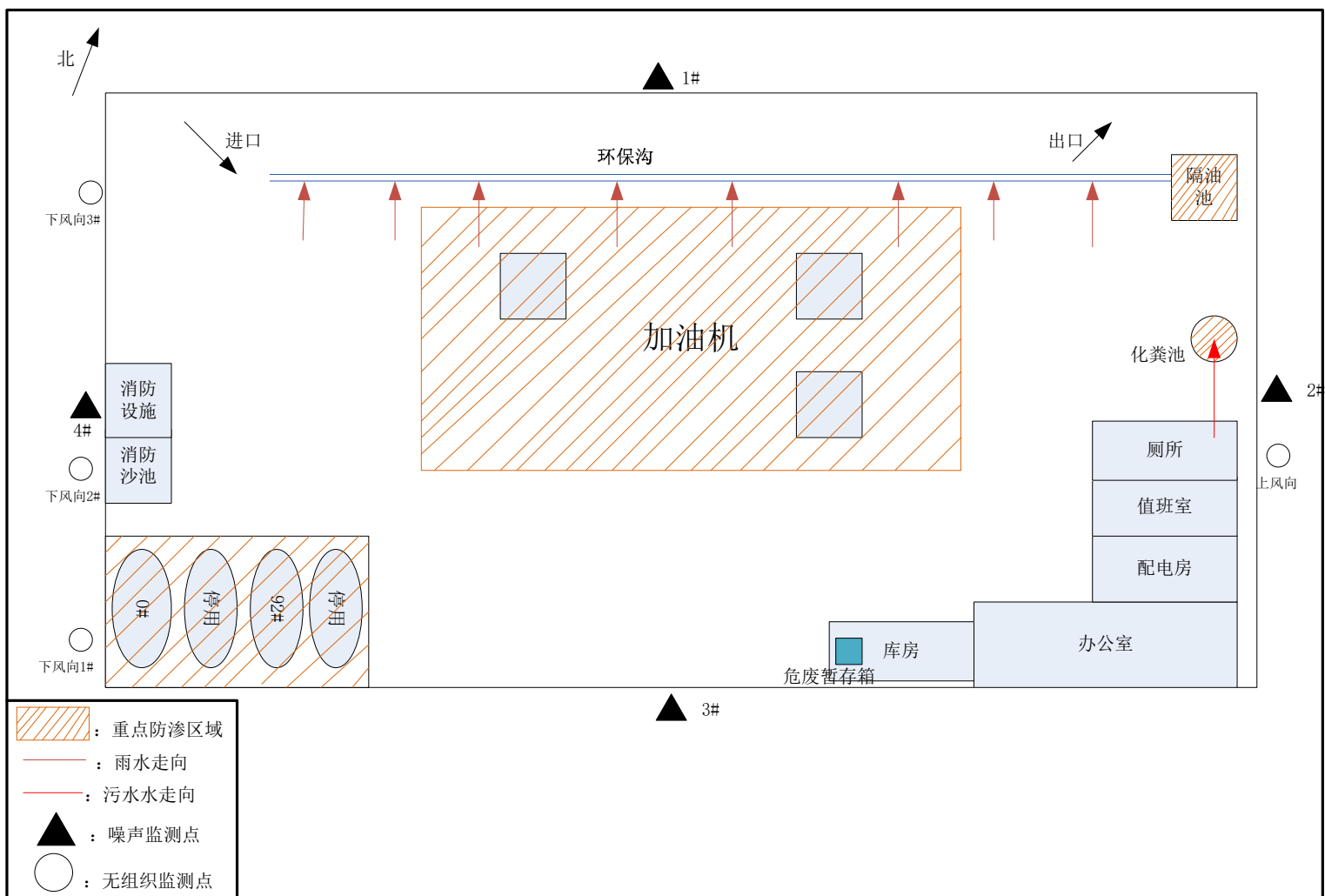
附图2 项目平面布置及监测布点图
