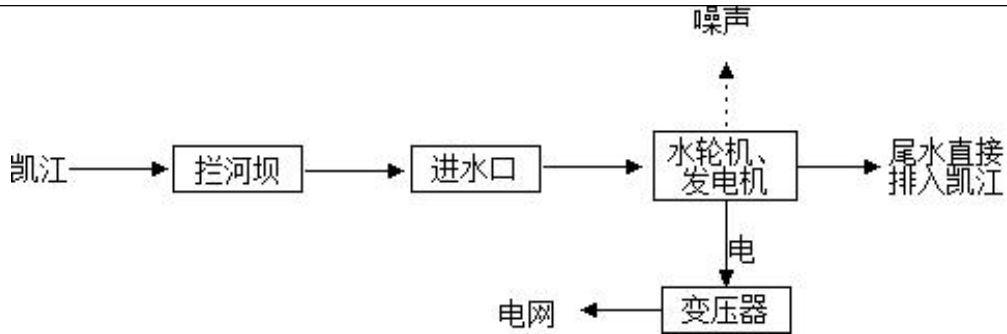
图4-2 发电工艺流程及产排污图
