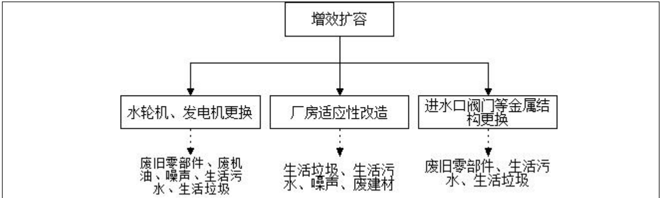
图4-1 增效扩容改造工艺流程及产排污图
