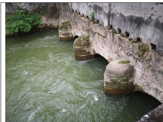
取水口
